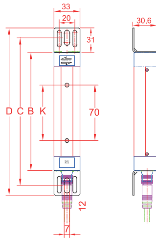
NC Dimensions
