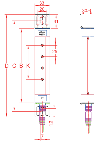
NB Dimensions
