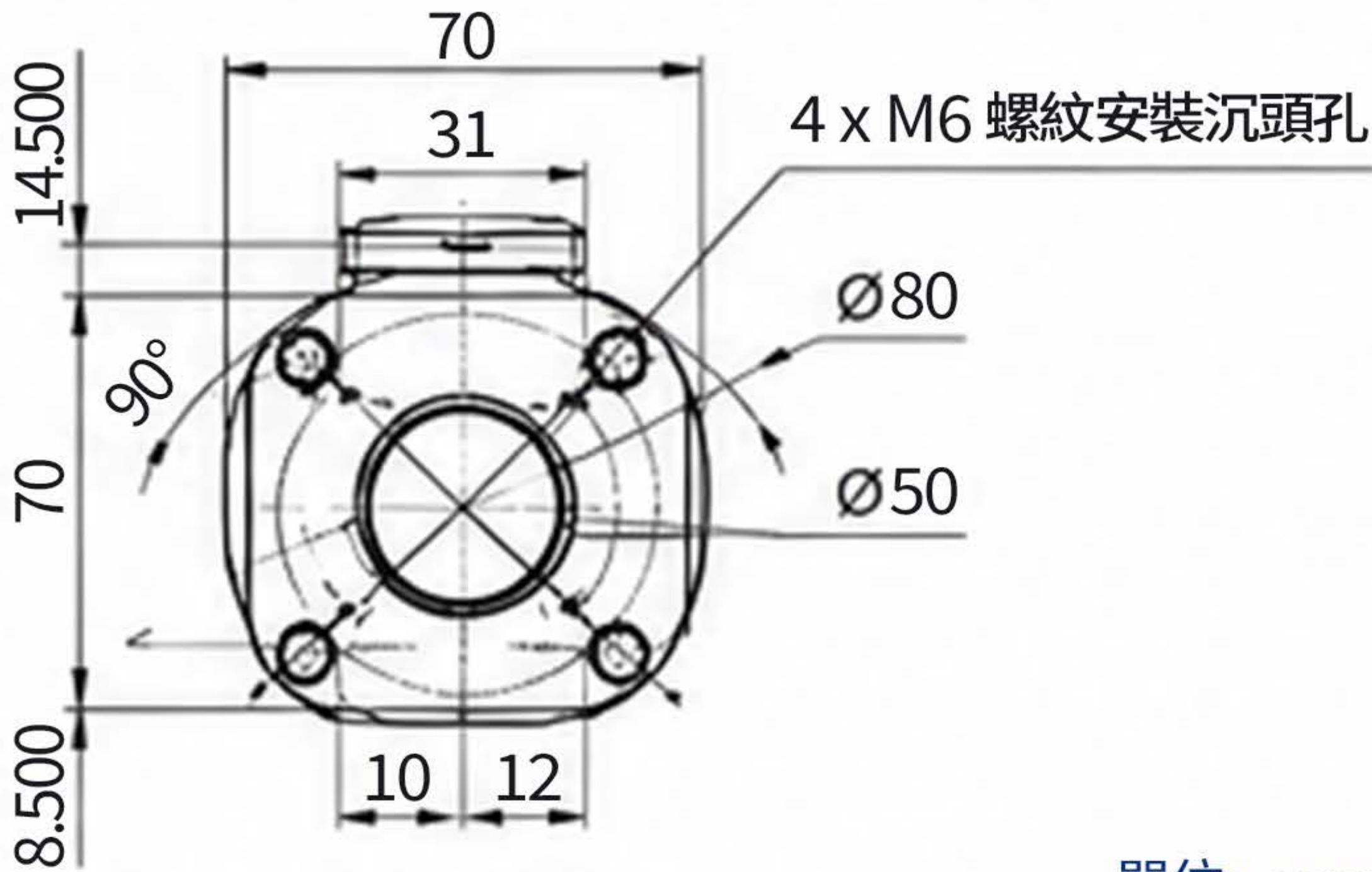
EQ-AQTT-10G 工具側 Tool Side
