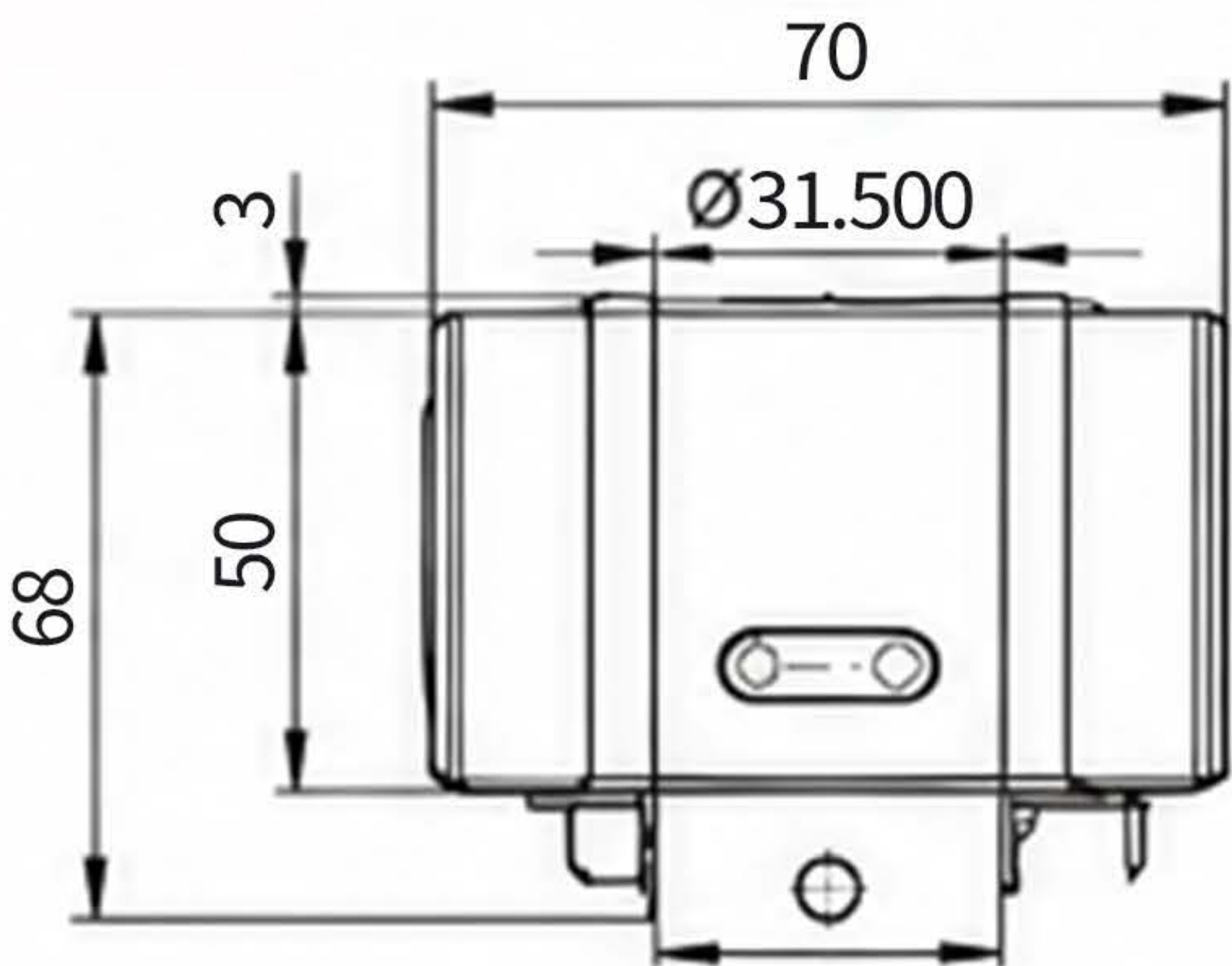
EQ-AQTR-10R 機器人側 Robot Side
