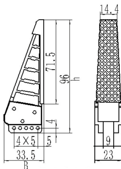
FAMR86 finger module
