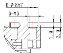
細部放大圖 B 比例 1 : 1
