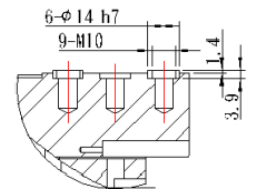
細部放大圖 B 比例 1 : 2
