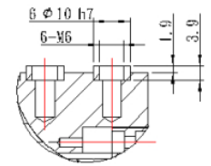
細部放大圖 B 比例 1 : 1
