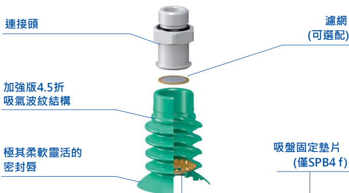
吸盤 SPB4/SPB4f 結構設計
